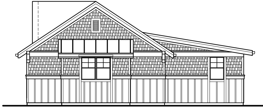
RIGHT ELEVATION
